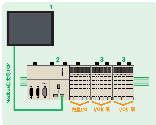
本地I/O
